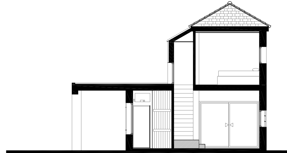
SECCIÓN A-A
