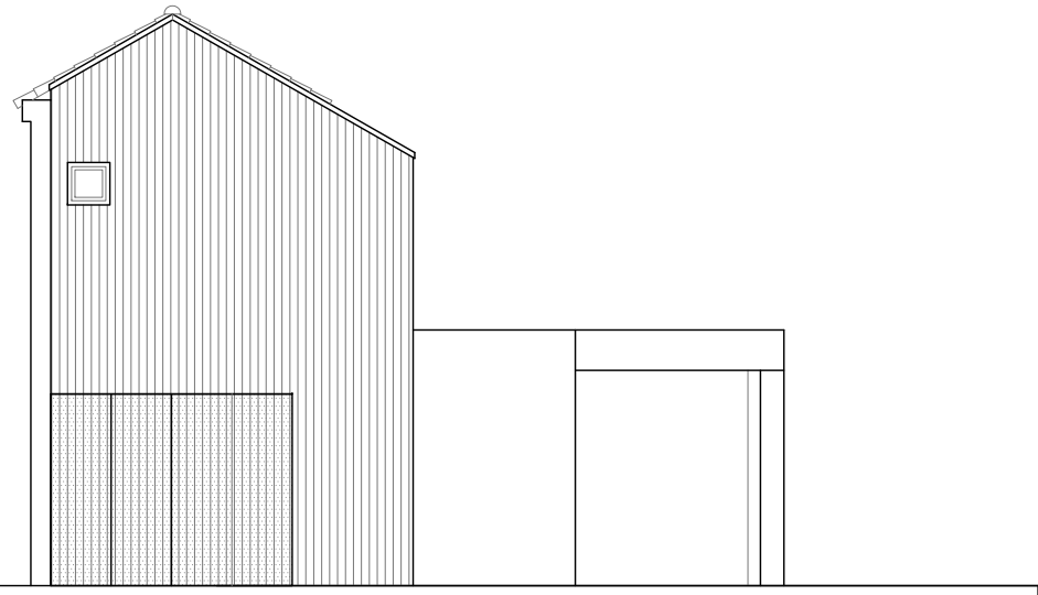
ALZADO SUR
