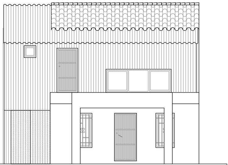
ALZADO ESTE
