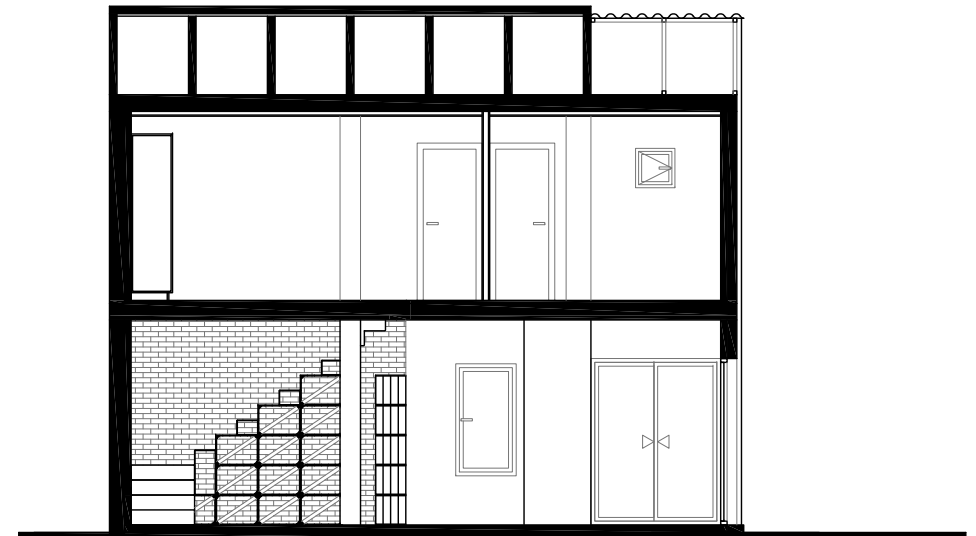
ALZADO B-B'
